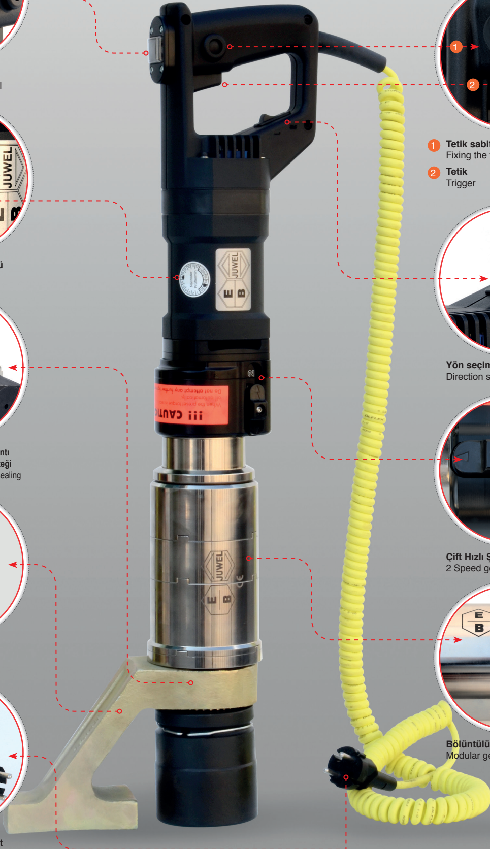
Çelik destek ayağı Steel angel reaction arm
