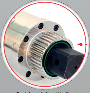
Destek ayağı frezeli bağlantı Yağ sızdırmazlık keçe desteği Reaction arm connection and sealing
